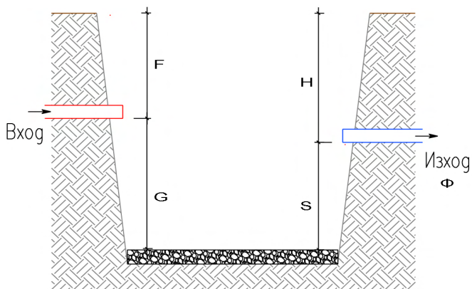
3. Полагане на входящ и изходящ тръбопровод до съоръжението
