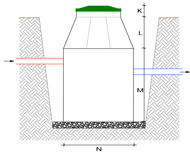
4. Монтаж на ПСОВ в изкопа
